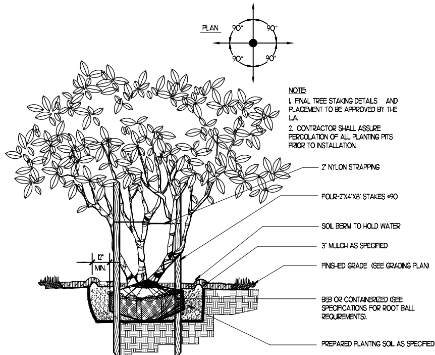
3 MULTI-TRUNK TREE SECTION DL\118018\5.dwg SCALE: N.T.S.
